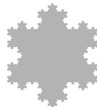
雪の結晶のようなフラクタル図形
